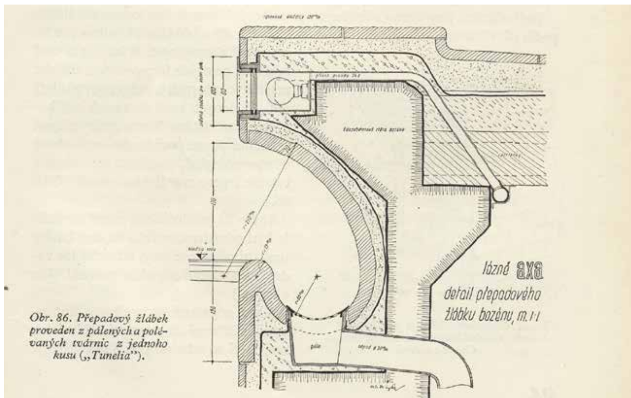
Obr. 15: Detail přepadového žlábku (převzato z: HOFBAUER, Alexander a KOLÁTOR, Václav. Lázně, stavba lázní, koupališť a plováren, jejich úprava a zařízení)
